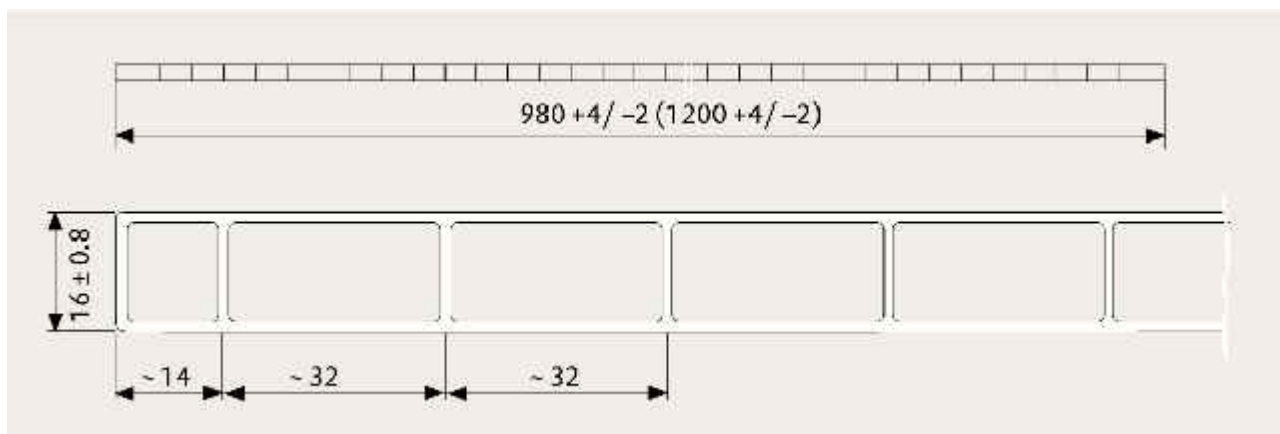
A PLEXIGLAS RESIST® SDP 16 metszete (a méretek mm-ben)
